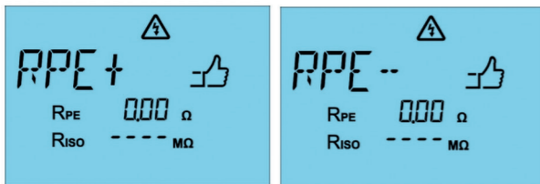
Abb. 56: R_{PE+} → positive Stromrichtung (links) und R_{PE-} → negative Stromrichtung (rechts)
