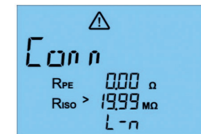
Abb. 45: Prüfung der Verbindung der stromführenden Leiter
