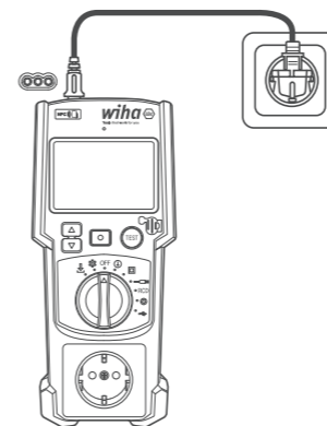
Abb. 9: Anschluss des Messgeräts an die Spannungsversorgung
