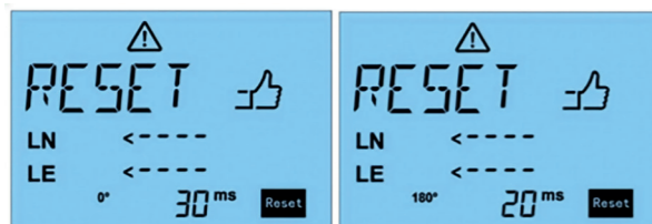
Abb. 52: Durchführung der RCD Messung mit 0° und 180°
