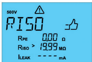
Abb. 20: Bestandene Isolationsprüfung
