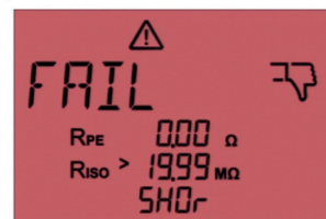
Abb. 48: Nicht bestandene Messung. Im Display wird „SHOr“ angezeigt. Kurzschluss zwischen L und N
