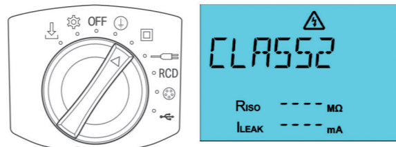
Abb. 27: Stellung des Drehschalters Displayanzeige
