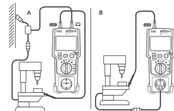
Abb. 55: Anschluss des Prüflings am Messgerät Option A: aktiver Messadapter Option B: passiver Messadapter
