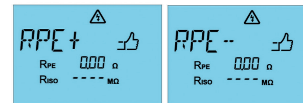
Abb. 39: R_{PE+} positive Stromrichtung (links) und R_{PE-} negative Stromrichtung (rechts)
