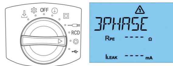
Abb. 54: Stellung des Drehschalters Displayanzeige
