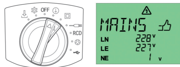
Abb. 8: Stellung des Drehschalters
