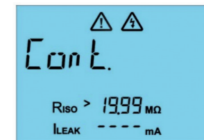
Abb. 34: Dauermessung (Cont. Modus)
