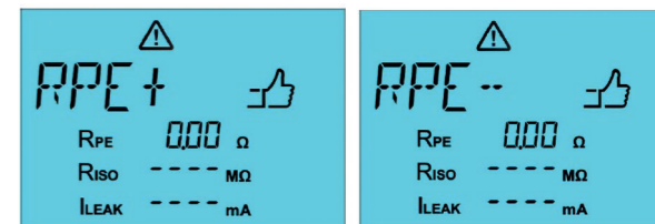
Abb. 14: R_{PE+} → positive Stromrichtung (links); R_{PE-} → negative Stromrichtung (rechts)
